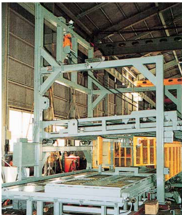
ブランク材ストック設備
